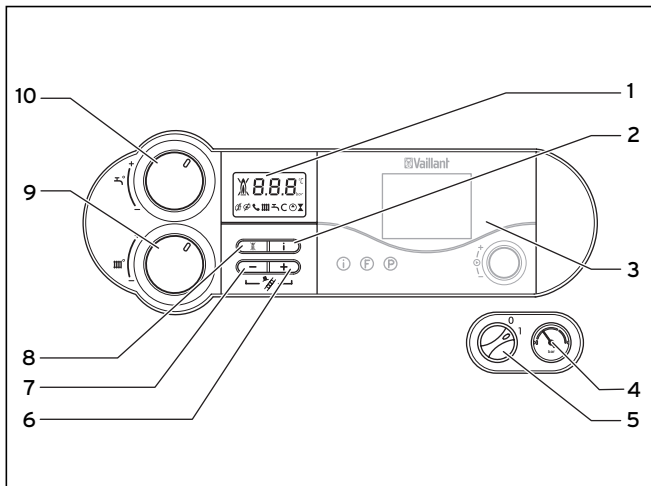
Abb. 4.3 Bedienelemente bei atmoTEC plus/turboTEC plus
